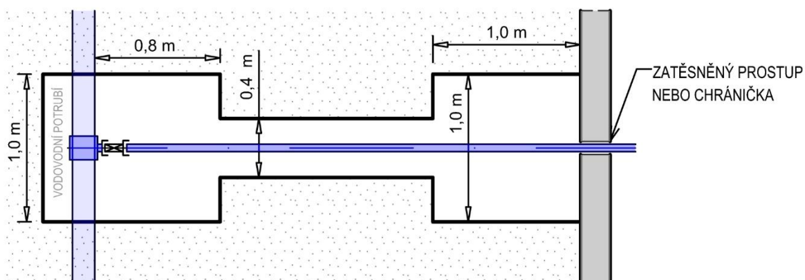
PŮDORYS - ROZMĚRY VÝKOPU
